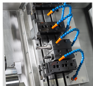
Sistema Gang Tools para portaherramientas: inclinación de 60°, fácil acceso del operador a los portaherramientas y evacuación de virutas.
